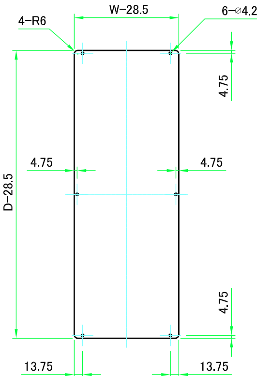
パネル裏面 / Panel Backside
