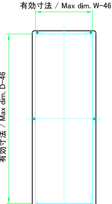
パネル表面 / Panel Frontside
